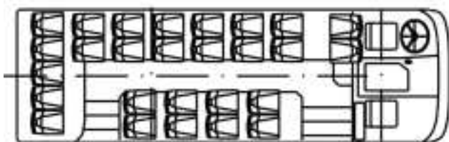
МАЗ 256200/270
