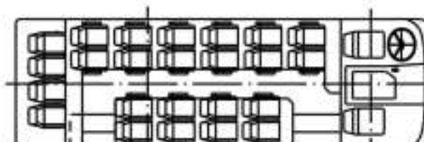
МАЗ 256100/170
